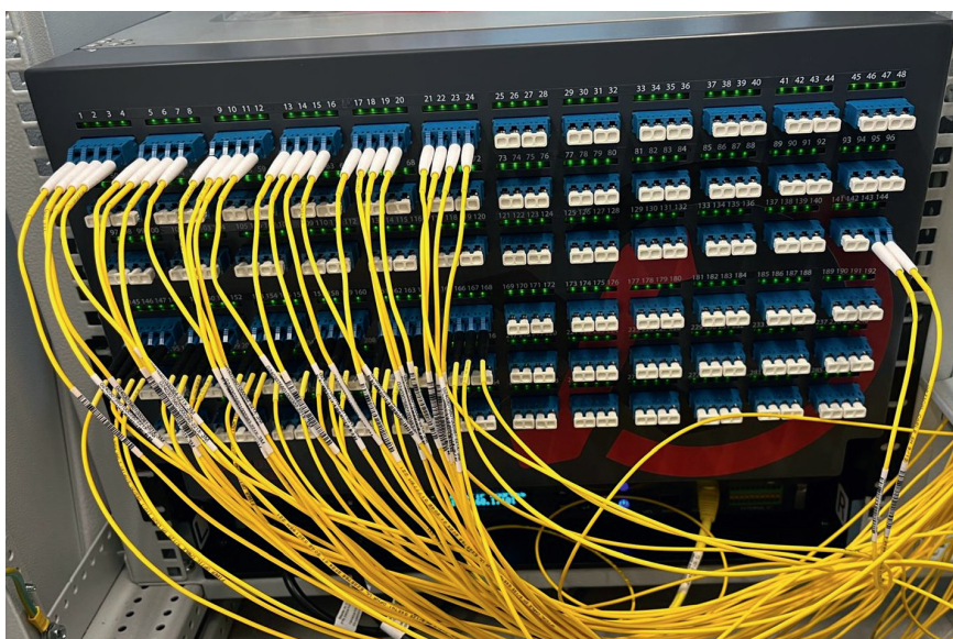
Die optische Matrix wird aktuell in einem Glasfaser-Ausbauprojekt im niederösterreichischen Waldviertel eingesetzt. 14 mit den Matrixen ausgerüstete POPs werden dort Open Access ermöglichen.
